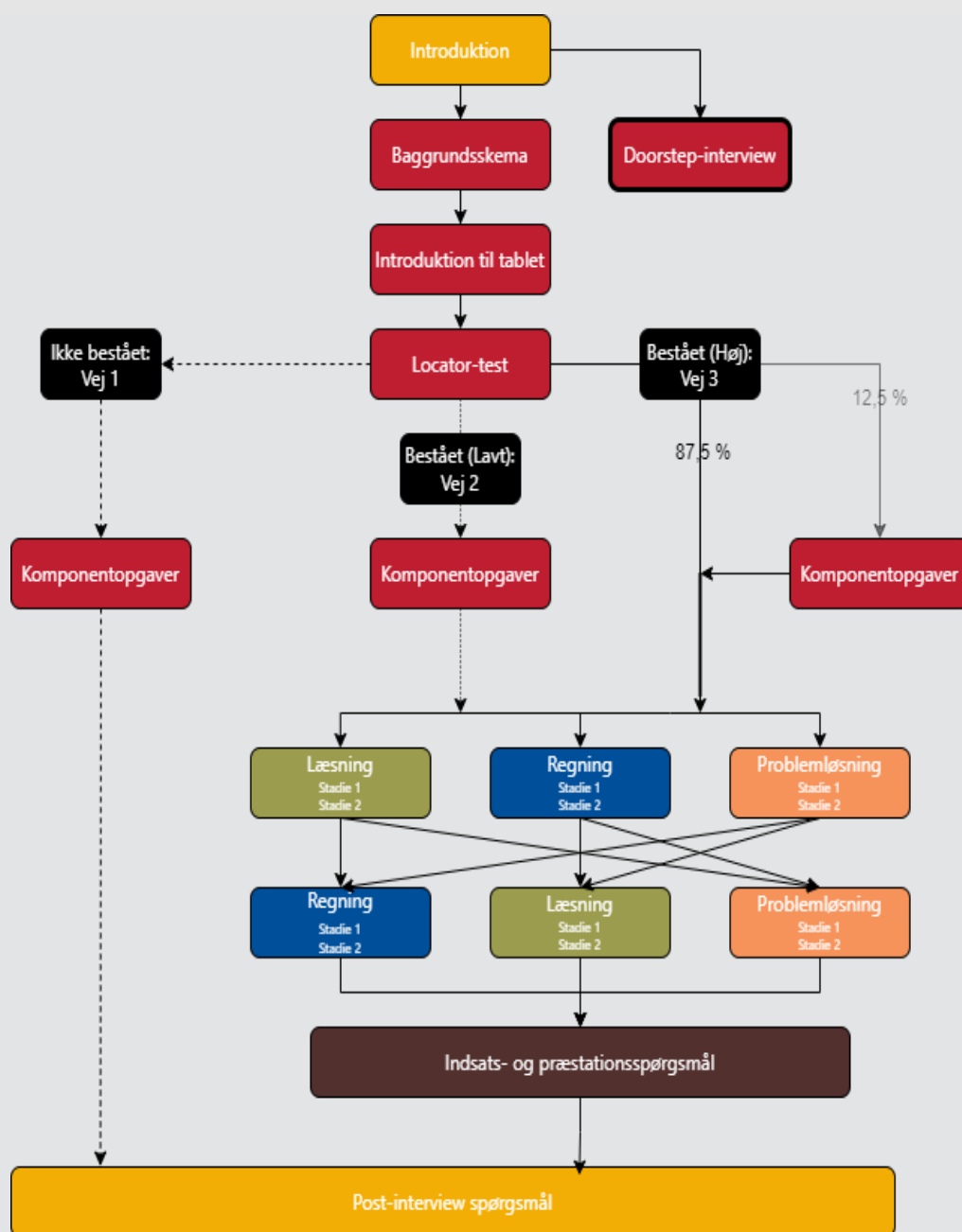
Figur 9.1 Dataindsamlingens forløb
